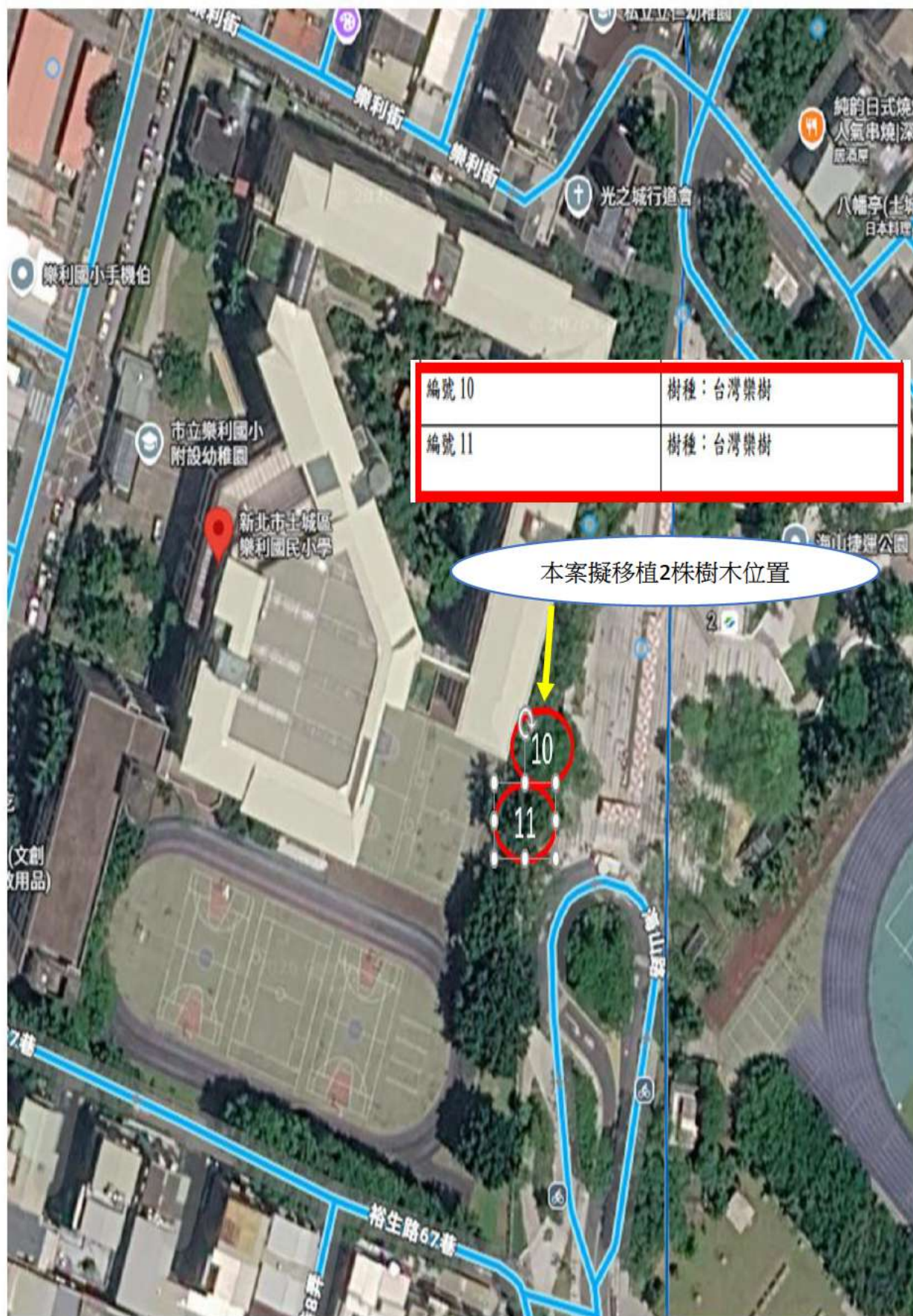
圖7 本案擬移植樹木編號及位置圖
